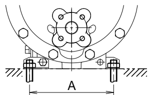
地脚螺栓的 固定位置
