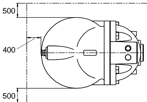
检修间距
