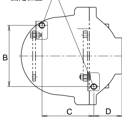
地脚螺栓的 固定位置
