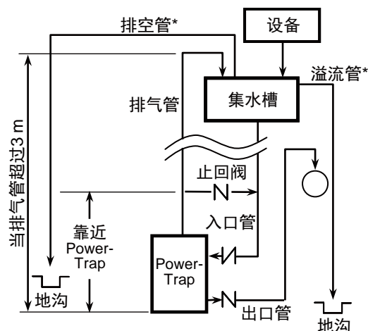
见图 2: 开放式 & 封闭式系统 *只是针对开放式回收系统
