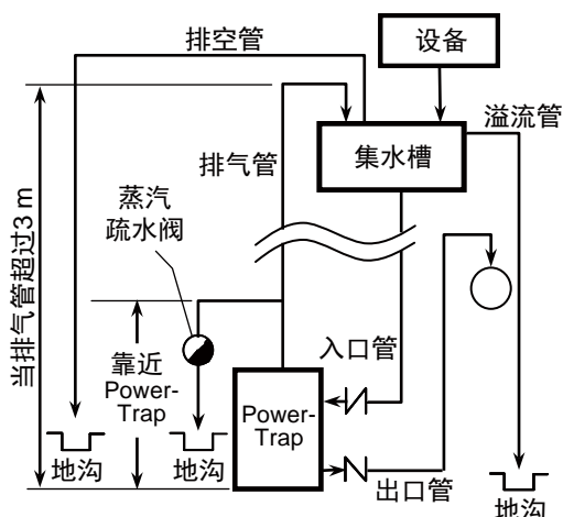
见图 1: 开放式系统
