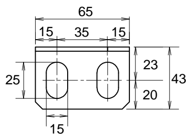
地脚螺栓定位架组件详细图
